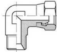
GOMITO M - F.GIR. CIL BSP 60°
