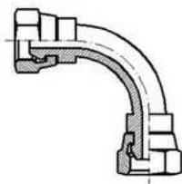
ADATTATORE 90° F.GIR. - F.GIR. BSP 60°
