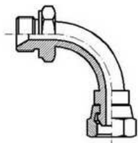
ADATTATORE 90° M - F.GIR BSP 60°
