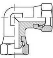
GOMITO F.GIR. - F.GIR. BSP 60°
