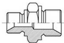
NIPPLLO RID. M - M CILINDRICO BSP CONO 60°
