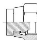
TAPPO FEMMINA GIR. BSP 60°
