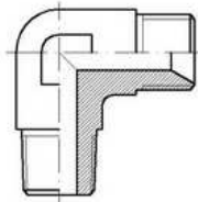
GOMITO M - M CIL. BSP 60° - CONICO
