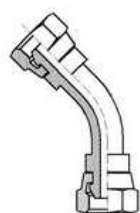
ADATTATORE 45° F.GIR. - F.GIR. BSP 60°
