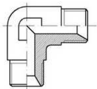
GOMITO M - M CIL. BSP 60°
