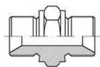
NIPPLLO M - M CILINDRICO BSP CONO 60°
